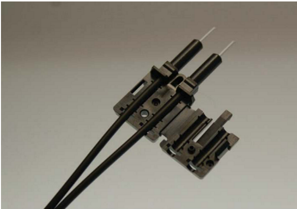
Abb. 55: In den Steckverbinder eingelegtes Kabel
