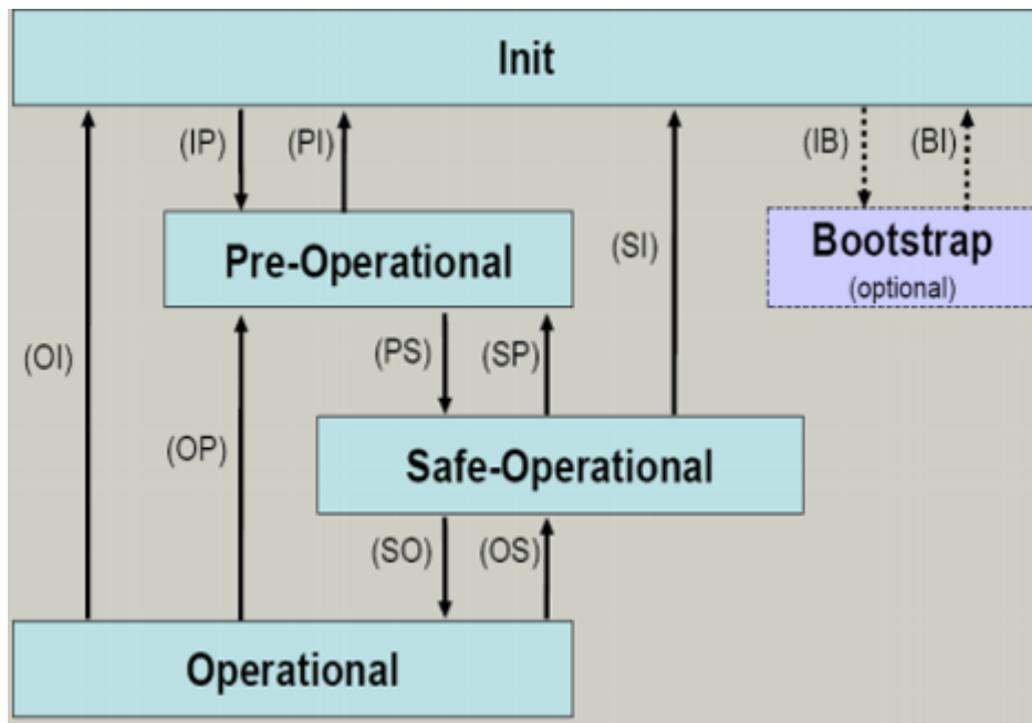
Abb. 26: Zustände der EtherCAT State Machine
