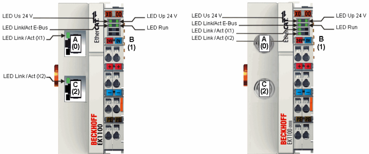
Abb. 24: Beispiel EtherCAT-Koppler EK1100 bzw. EK1100-0008 mit 3 Ports
