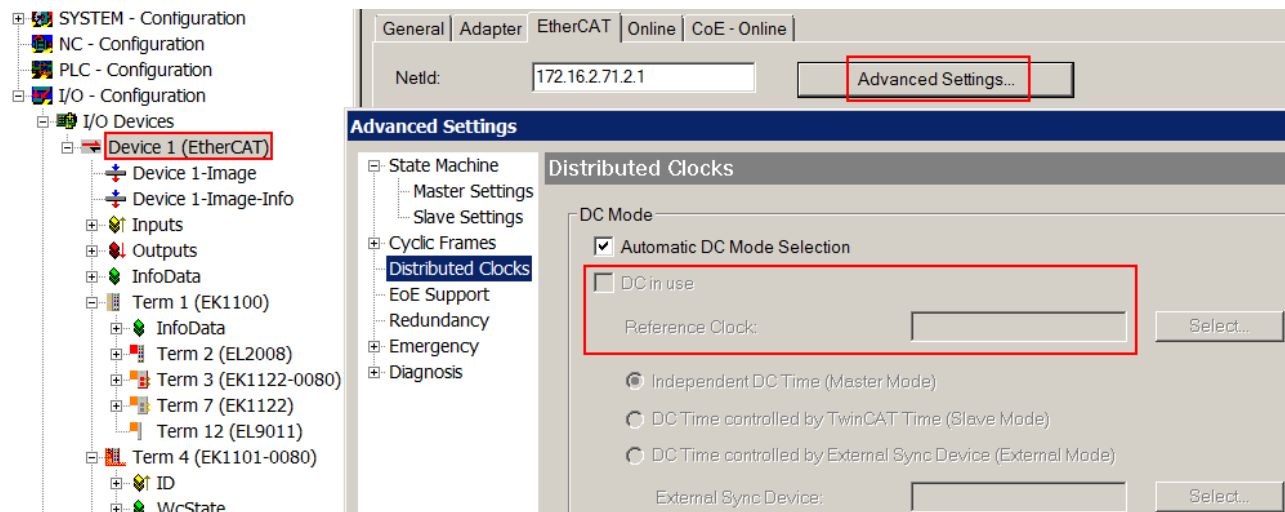
Abb. 17: DC-Master-Einstellung
