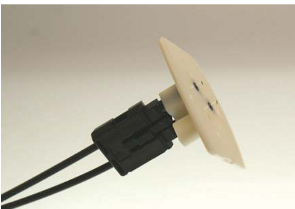
Abb. 58: Schleiflehre mit herausragenden Faserenden
