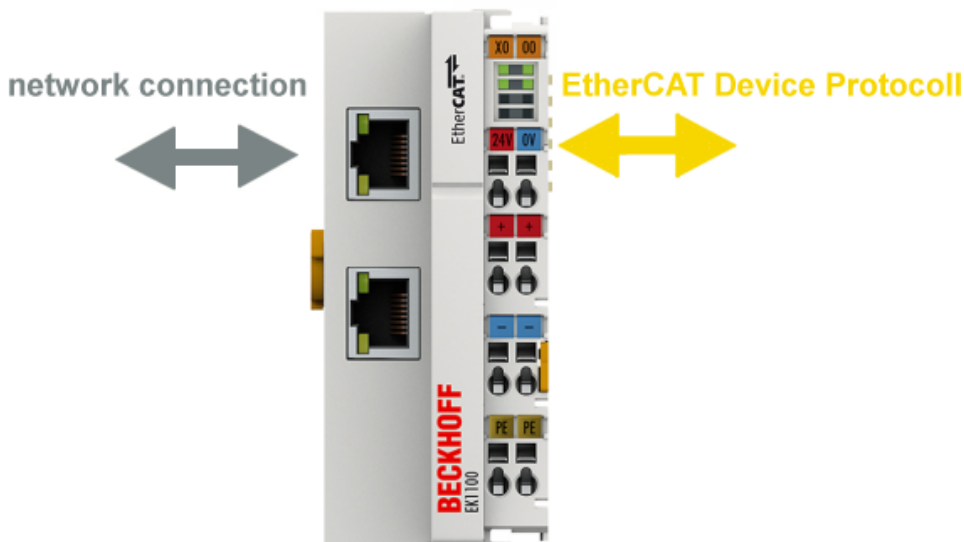
Abb. 4: Kommunikationsschema EtherCAT-Koppler
