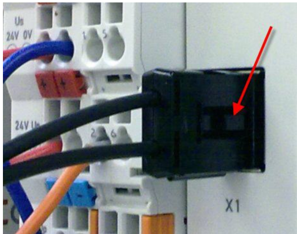
Abb. 52: Rastnase mit Entriegelung am POF-Duplex-Stecker
