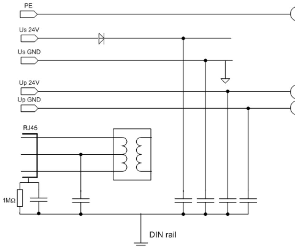
Abb. 45: Erdungskonzept EKxxxx
