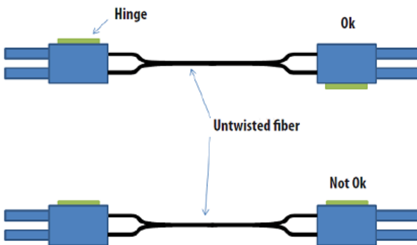
Abb. 57: Korrekt verbundene Optische Kanäle
