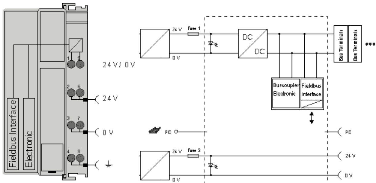
Abb. 44: Potenzialschaltbild EKxxxx
