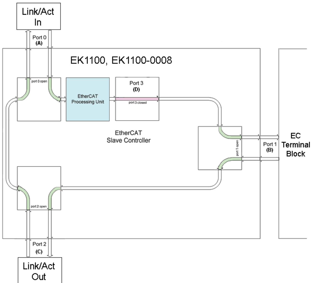
Abb. 25: Interne und externe Port-Zuordnung Buskoppler EK1100 bzw. EK1100-0008
