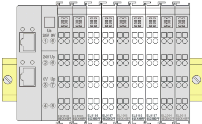
Abb. 46: Korrekte Positionierung
