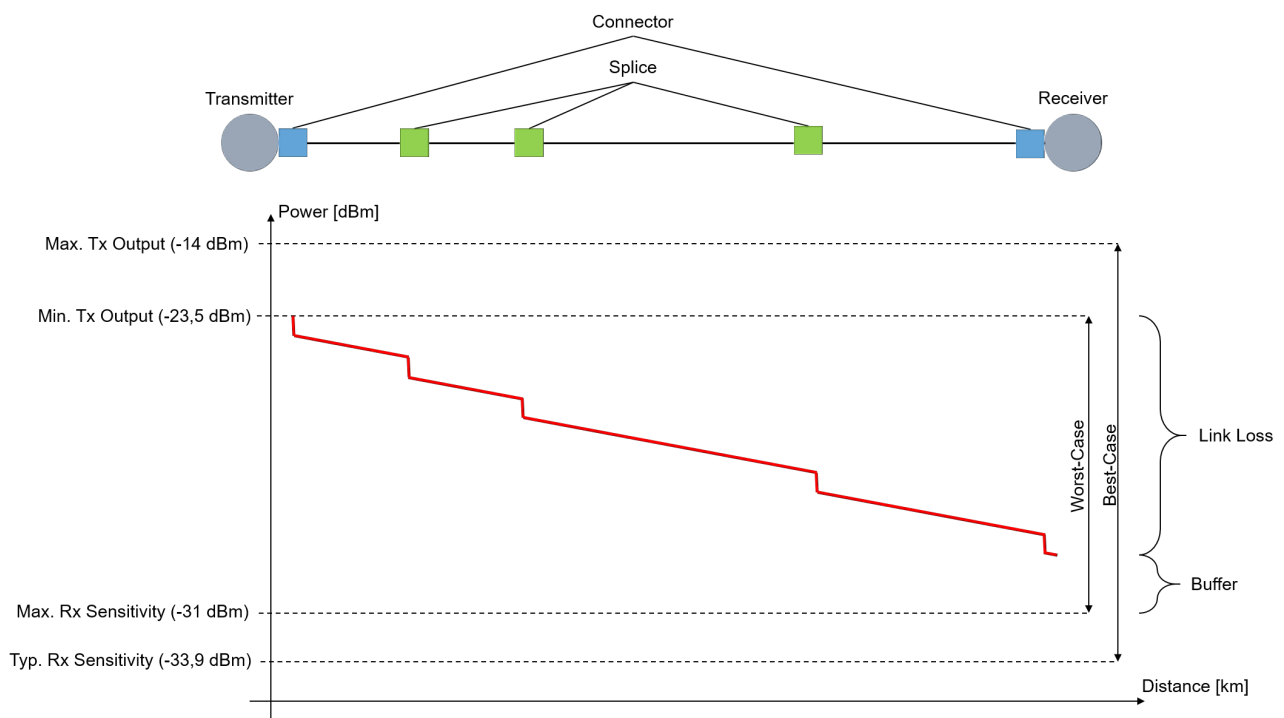
Abb. 50: Leistungs- und Dämpfungsbudget
