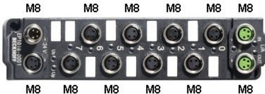
Abb. 43: EtherCAT Box mit M8-Steckverbindern
