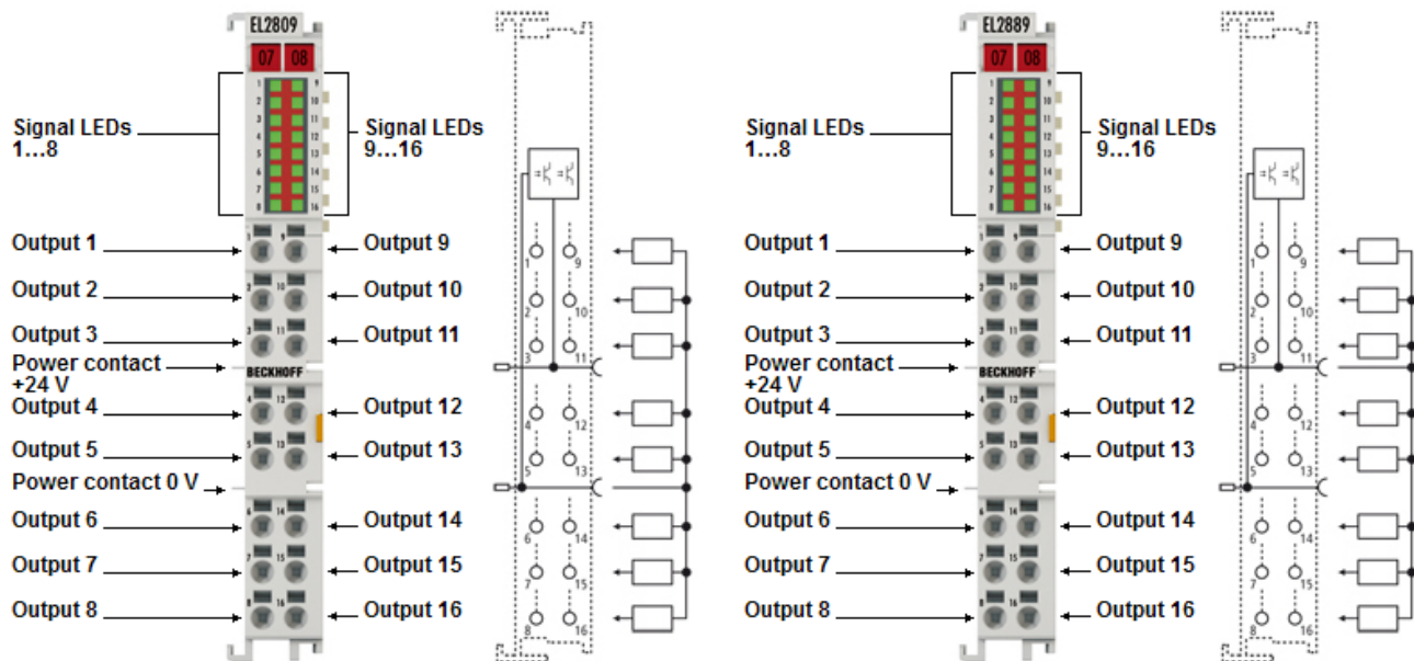
Abb. 11: EL2809, EL2889
