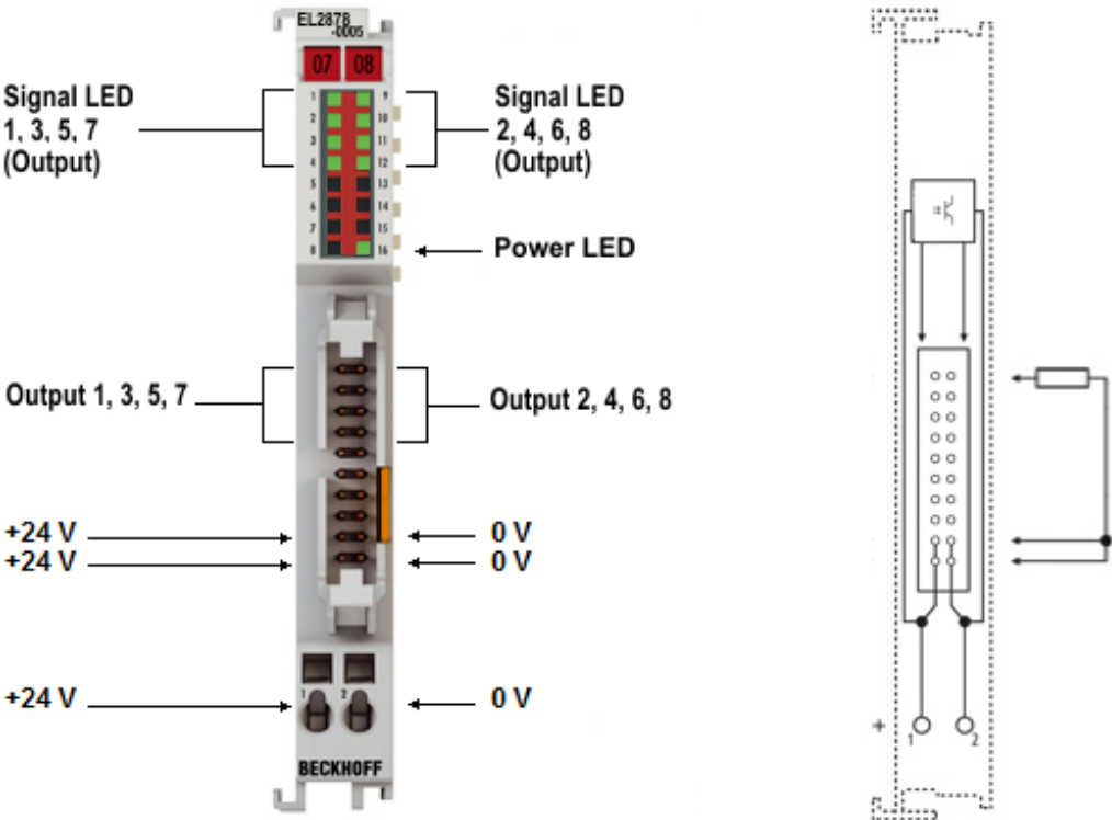
Abb. 28: EL2878-0005
