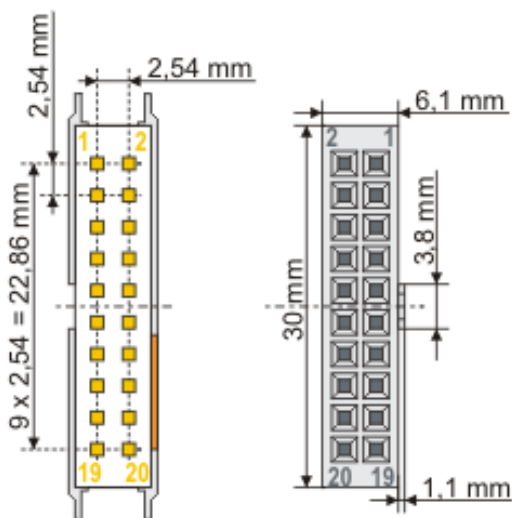
Abb. 26: Abmessungen der 20-poligen Stiftleiste der Klemme und der passenden Federleiste, Beschriftung siehe Kontaktbelegung
