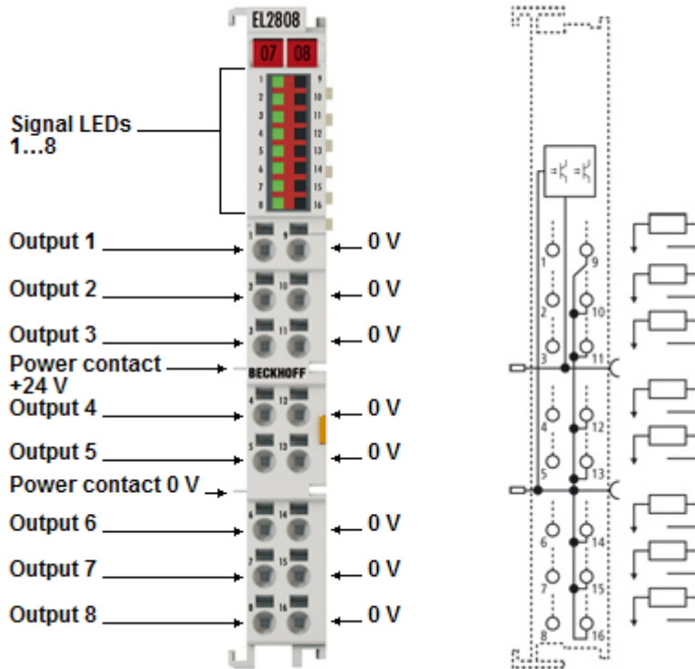
Abb. 7: EL2808
