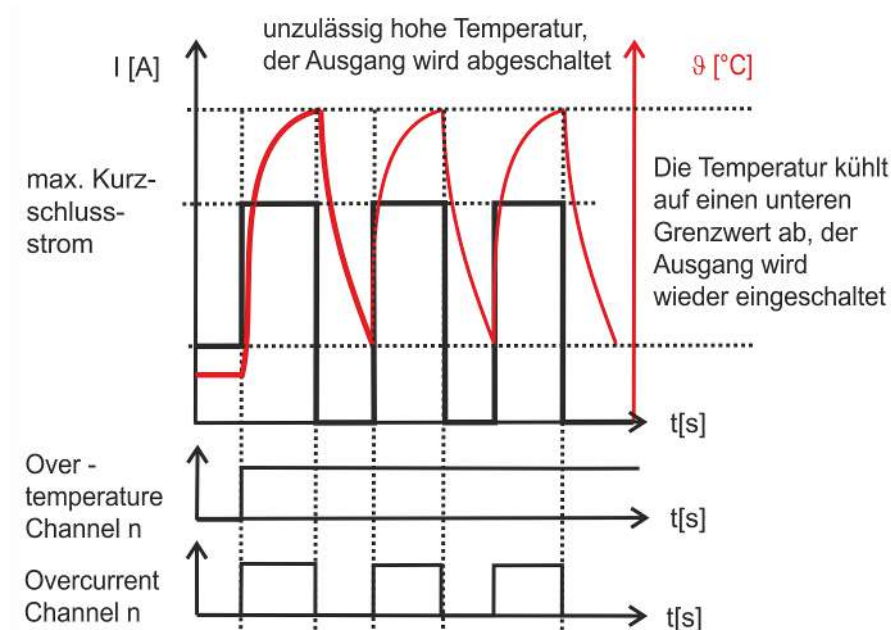
Abb. 16: Schematische Darstellung der thermischen Abschaltung bei Überlast
