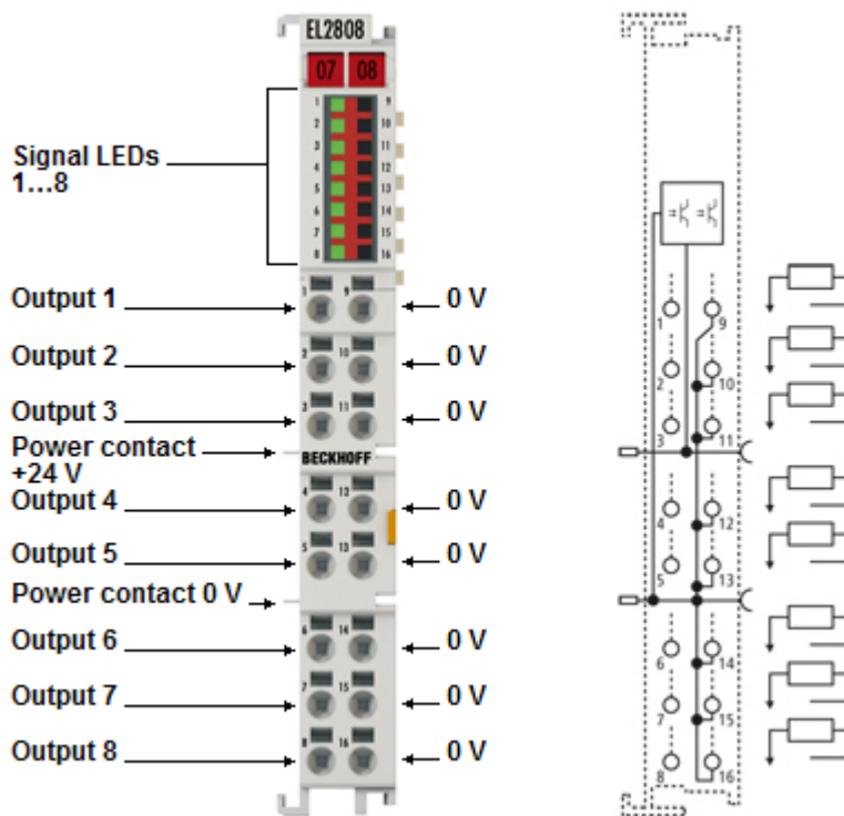
Abb. 8: EL2808
