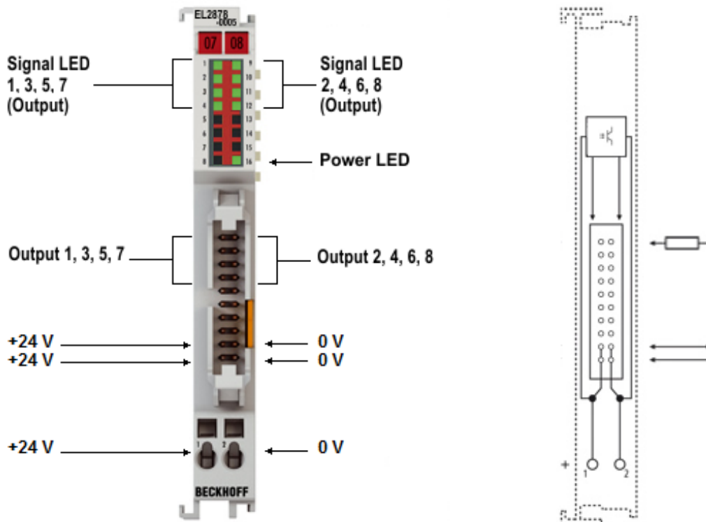
Abb. 27: EL2878-0005
