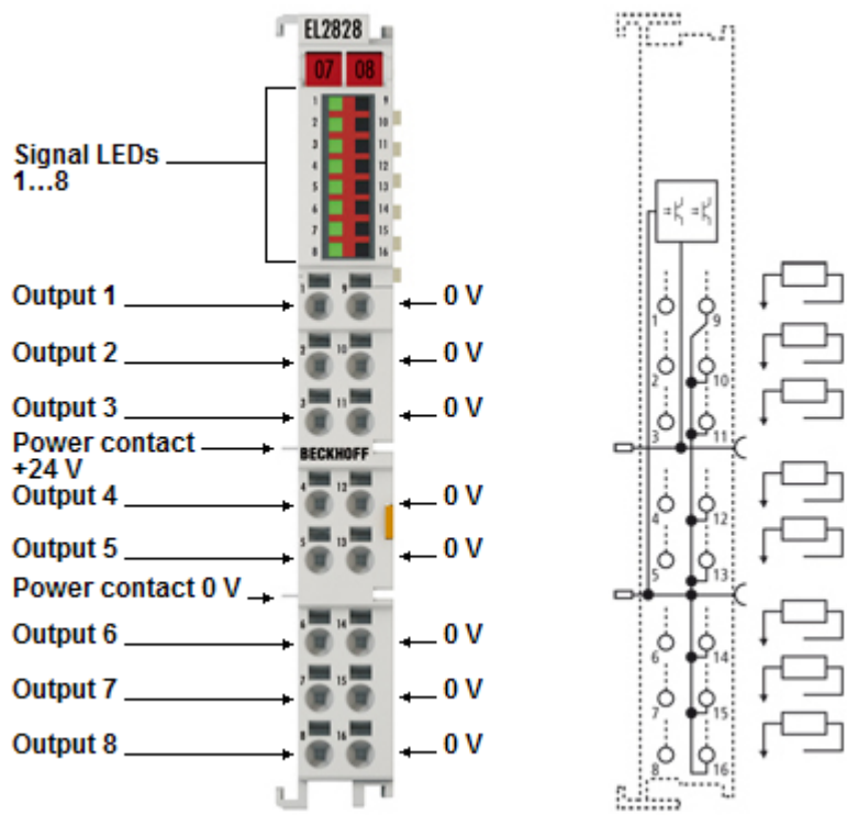
Abb. 10: EL2828
