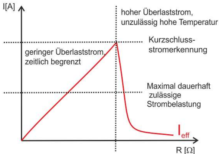
Abb. 15: Strombegrenzung bei Überlast
