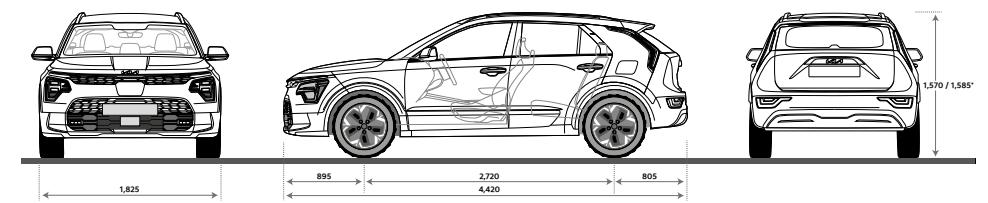
Masse EV (mm)
