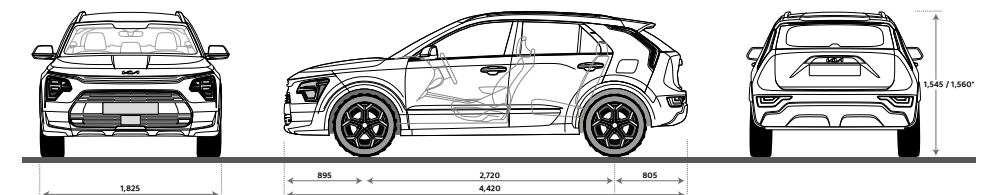
Masse HEV/PHEV (mm)
