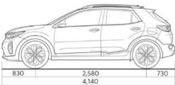
Dimensioni (mm) * Con mancorrenti sul tetto
